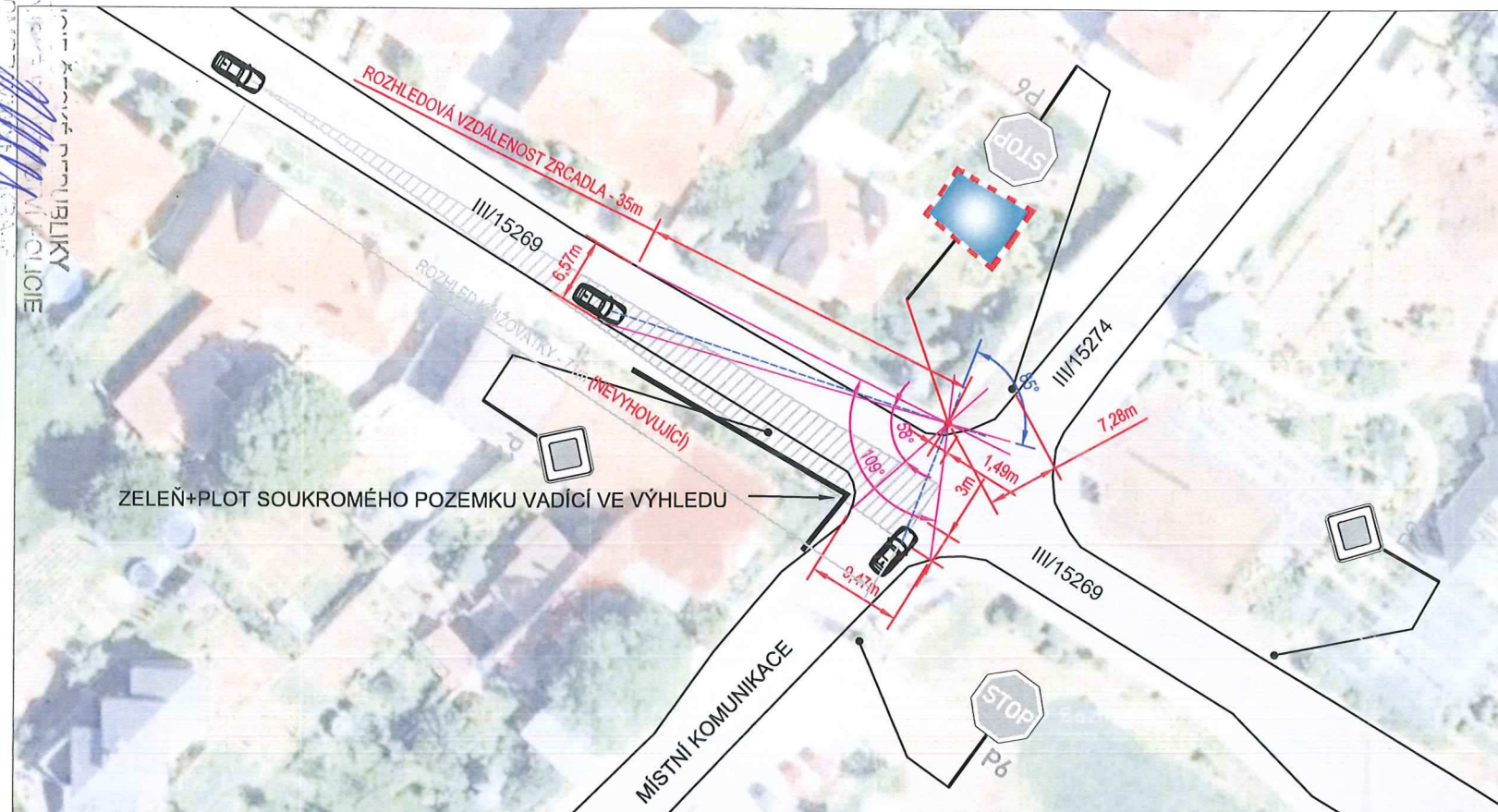
VÝHLED ŘIDIČE
