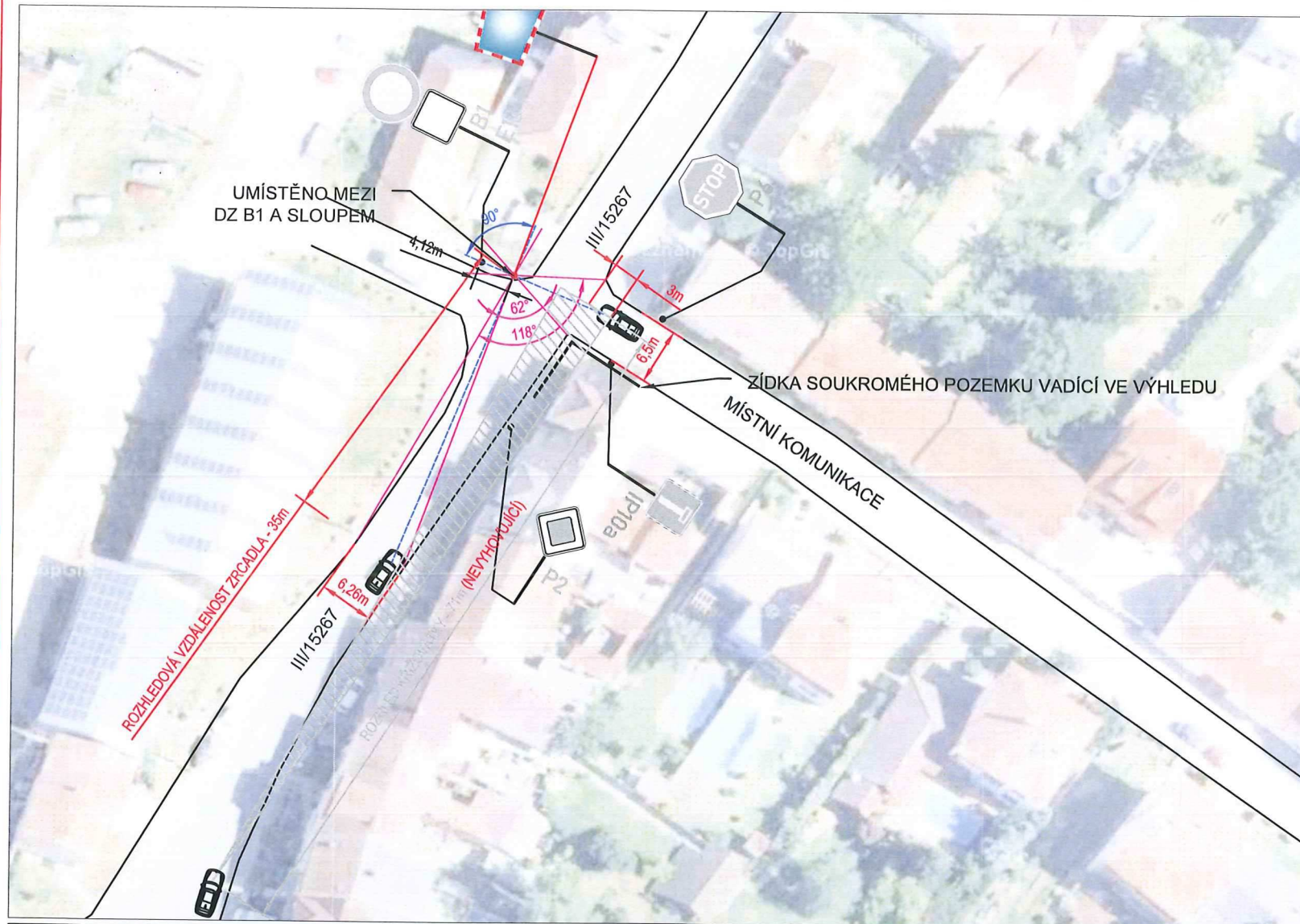
VÝHLED ŘIDIČE
